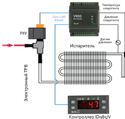
Схема типового использования с ID985/V Драйвер электронного TPB V800
