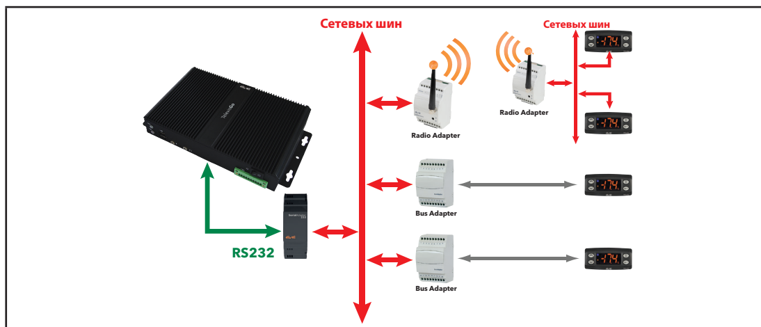
Пример сети со шлюзом RS232 / RS485
