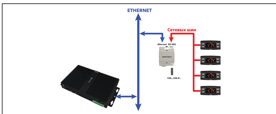
Пример сети со шлюзом Ethernet / RS485
